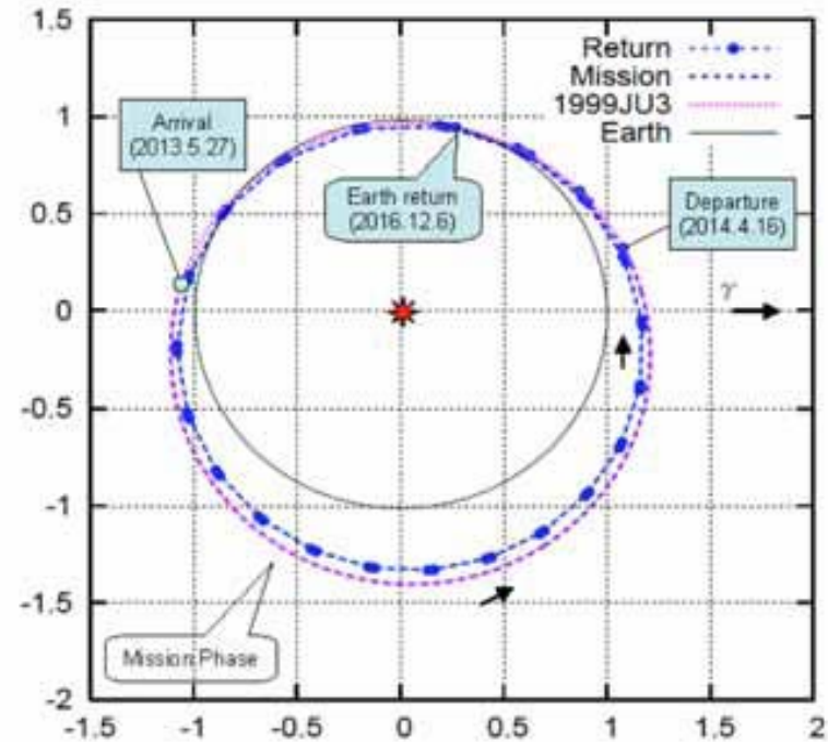
1999JU3到着～地球帰還
