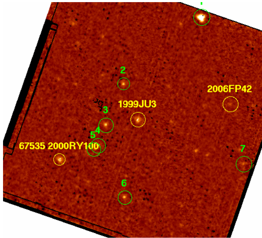
15 \mu mでの観測結果
