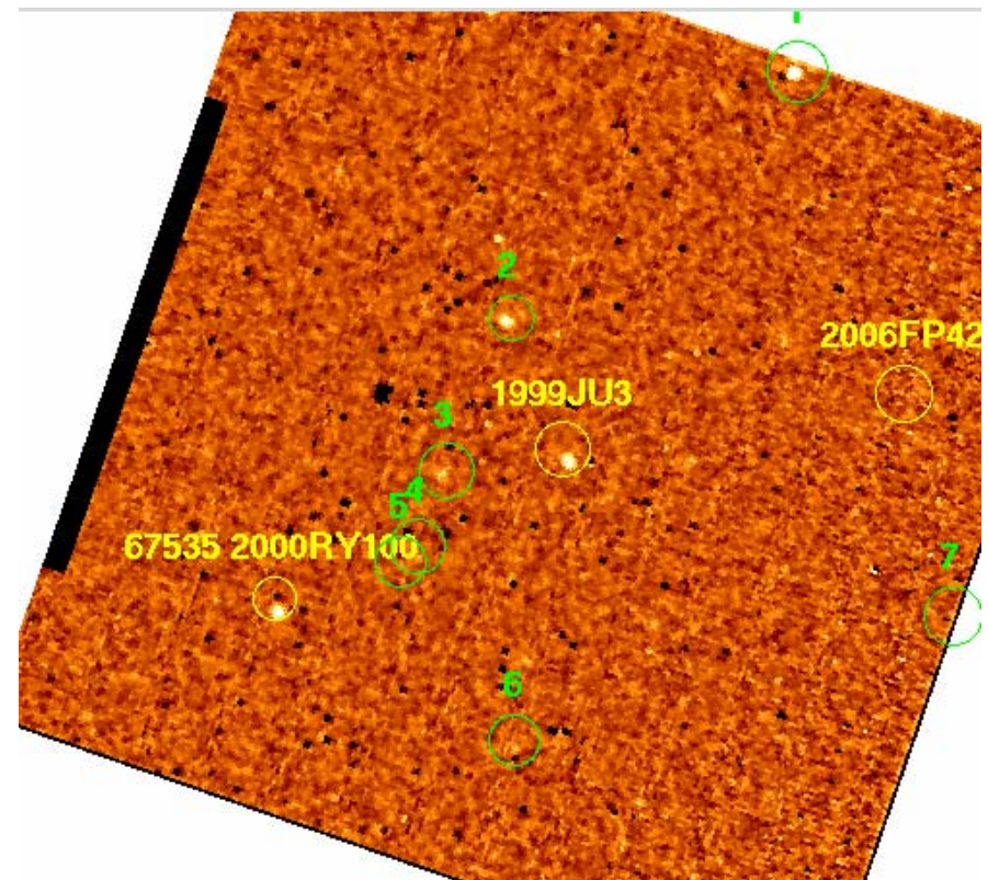
24 \mu mでの観測結果
