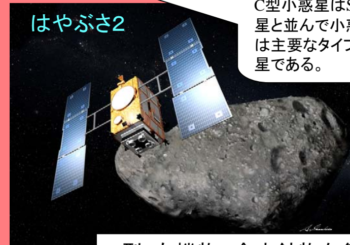
C型: 有機物、含水鉱物を多く含む
