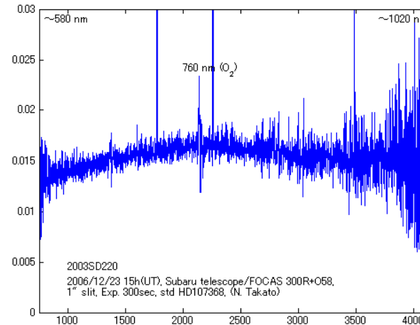
すばるFOCASを用いた2003SD220の可視スペクトル観測結果
