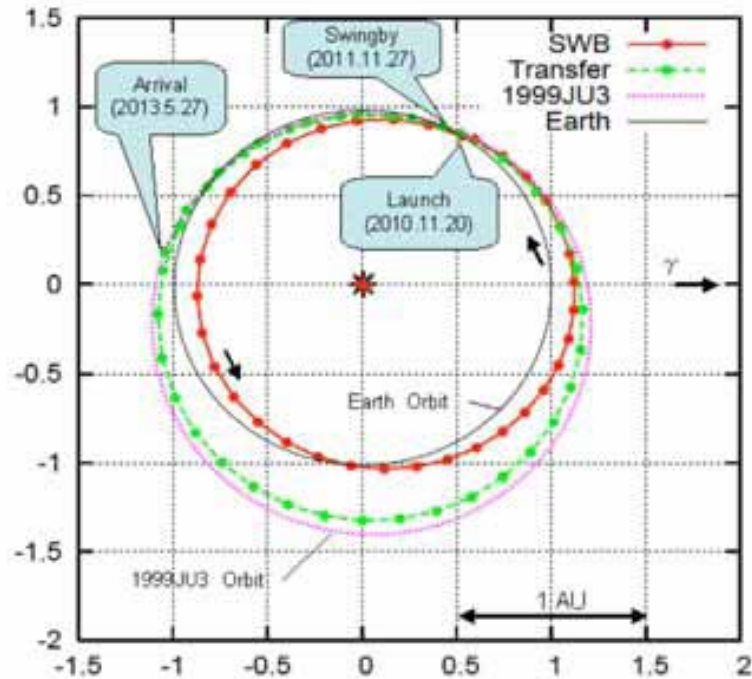
打ち上げ～1999JU3到着
