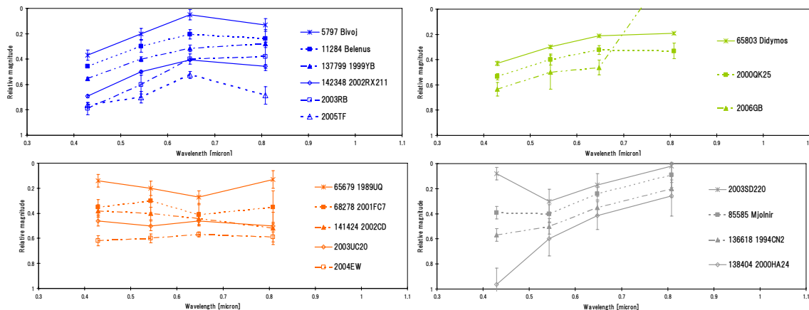
木曾・鹿林で取得した探査候補天体多色スペクトル
